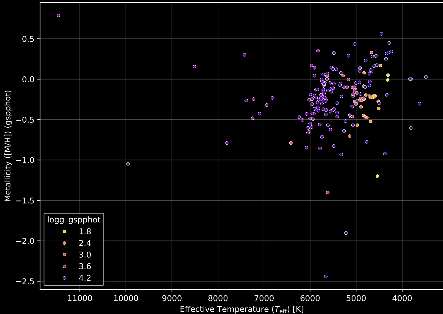
APOGEE DR17 Field: [198+41_MGA] Stellar Population Parameters (n= 191)
